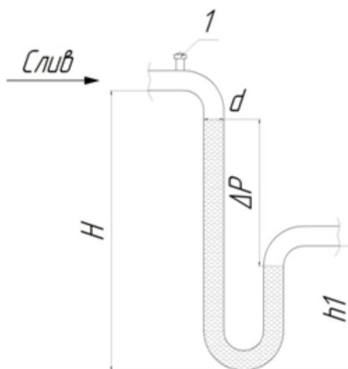
Рис. 3. Размеры трубопровода гидрозатвора в случае установки увлажнителя перед секцией вентилятора
