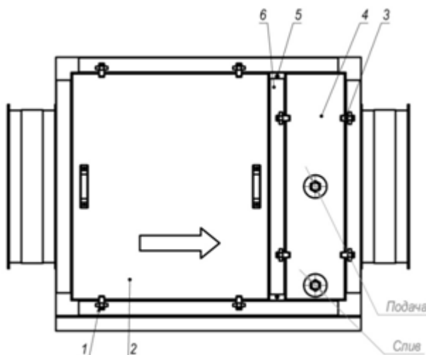
Рис. 6. Секция увлажнителя
